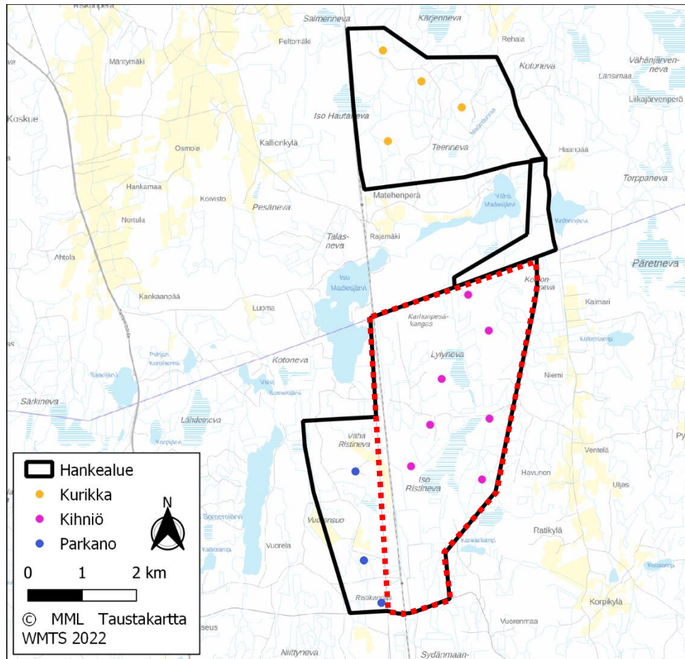
Kuva 3 YVA:n hankevaihtoehdon 1 (VE 1) alustava voimaloiden sijoitussuunnitelma. Kaava-alueen raja punaisella.
