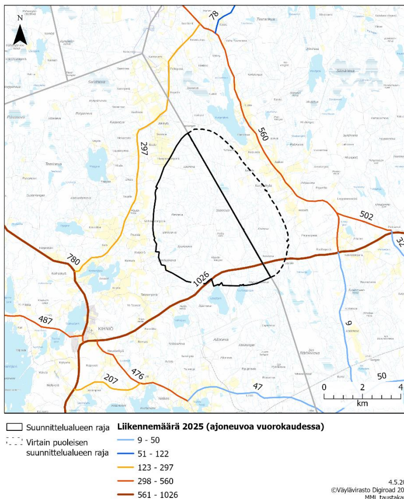
Kuva 3-2. Liikenneverkko ja keskimääräiset liikennemäärät suunnittelualan läheisyydessä.
