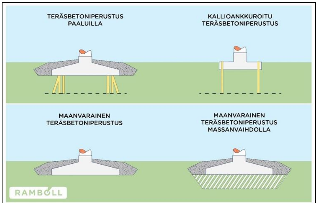
Kuva 2-5. Tuulivoimaloiden perustamistekniikoita.
