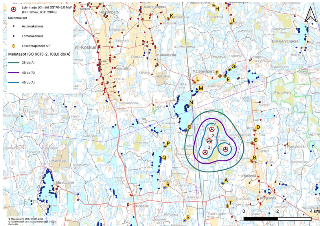
Kuva 1. Melumallinnuksen tulos Lylyharjun tuulivoimapaiston Kihniön alueelle suunnitellulla voimasijoittelulla.
