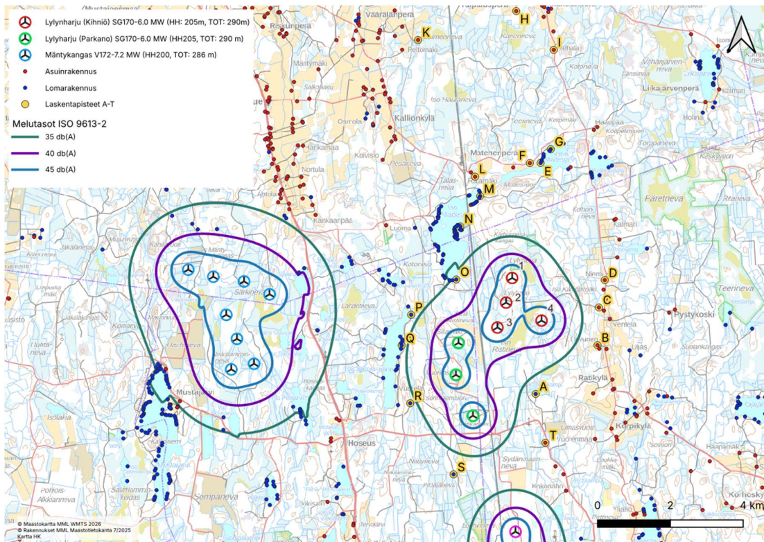
Kuva 2. Yhteismelumallinnuksen tulos, kun huomioidaan Lylyharjun tuulivoimapaiston kaikki suunnitellut voimalat sekä Mäntykankaan ja Mäntyperän tuulivoimahankkeiden suunnitellut voimalat.
