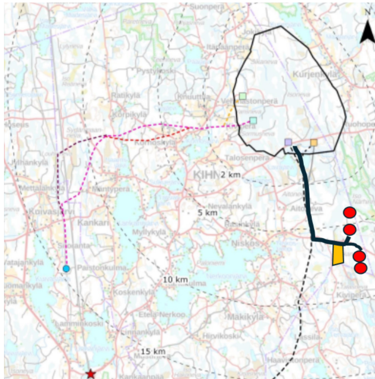
Kuva 45: Närhinkankaan (punaiset pallot voimaloita) liittyminen Myyräkankaan YVA:ssa esitettyyn sähkönsiirron linjausvaihtoehtoon.
