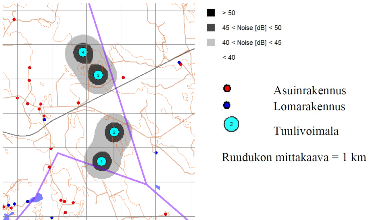
Kuva 28: Hankealueelle mahdollisella voimavaihtoehdolla tehty melumallinnus (106 dB)
